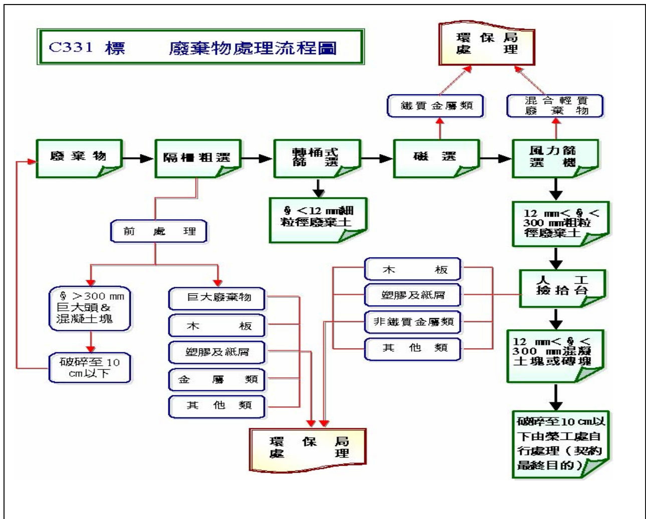
圖一 建築廢棄物再生處理流程圖
