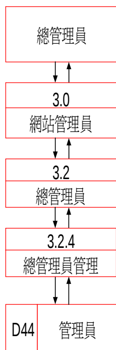
資料流程圖
