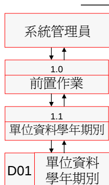
資料流程圖
