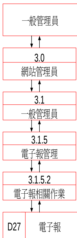
資料流程圖
