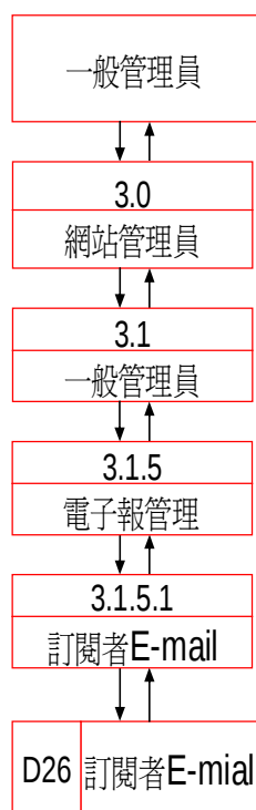
資料流程圖
