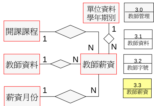
實體關係圖
