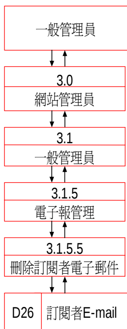
資料流程圖
