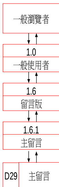
資料流程圖
