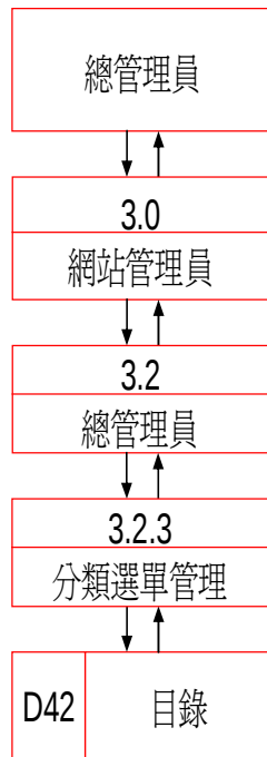
資料流程圖
