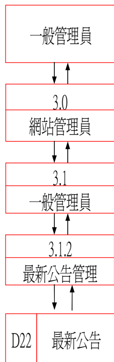
資料流程圖
