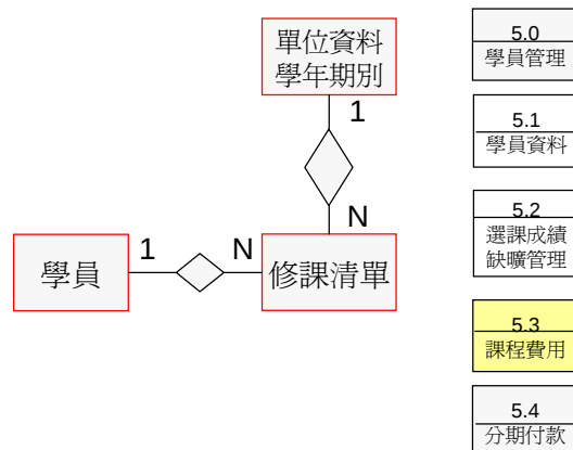
實體關係圖
