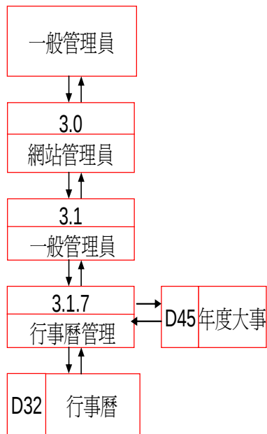
資料流程圖
