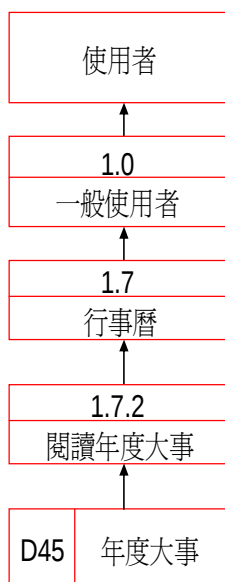
資料流程圖
