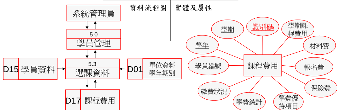
實體關係圖
