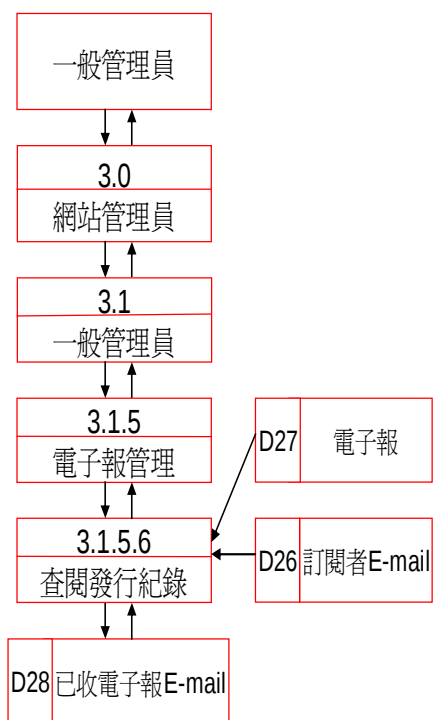
資料流程圖
