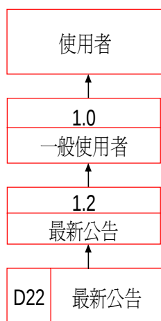
資料流程圖
