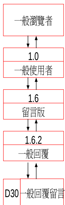
資料流程圖
