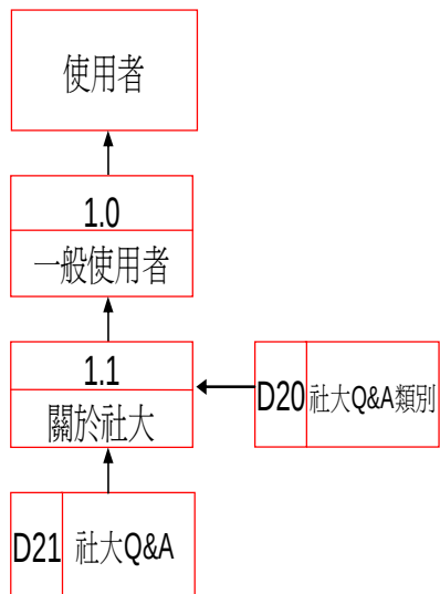
資料流程圖
