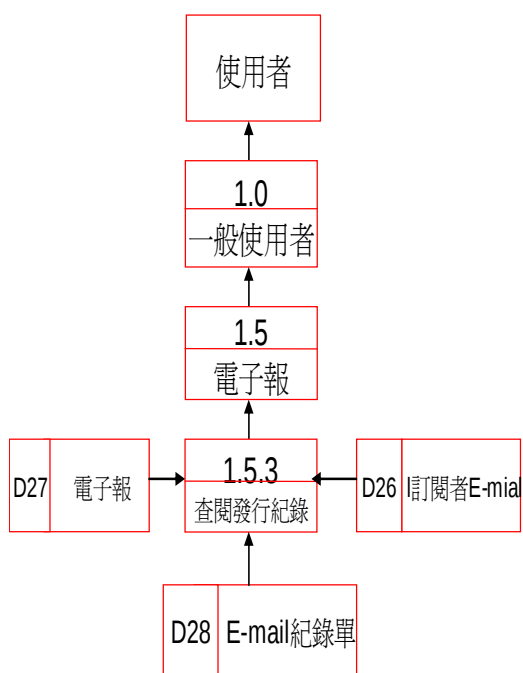
資料流程圖
