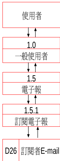
資料流程圖
