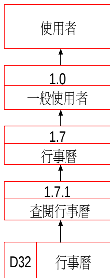
資料流程圖
