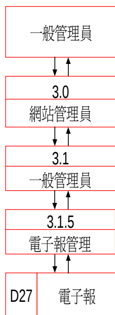
資料流程圖
