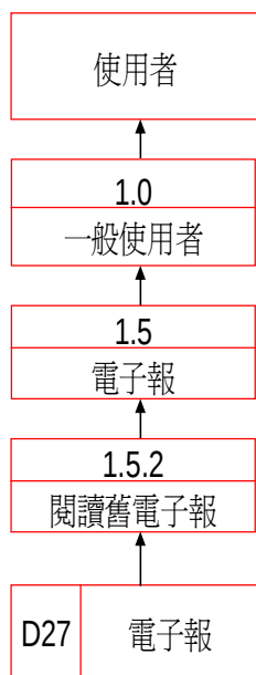
資料流程圖
