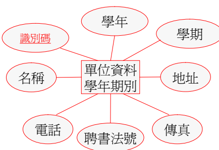
實體及屬性
