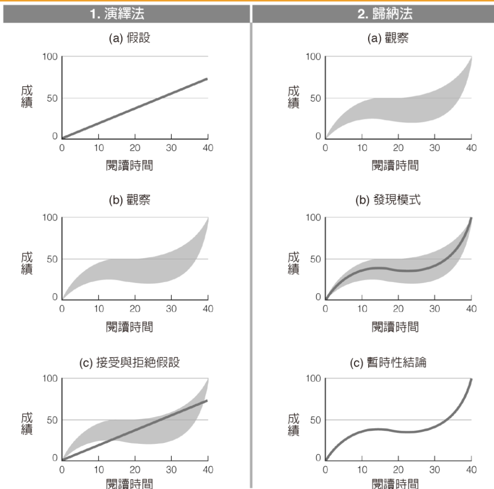
圖 2-3 演繹法與歸納法。
